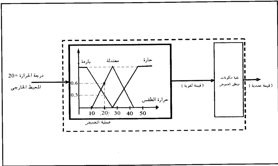
شكل (٥ - ٤) عملية التغميض وموقعها في النظام الغموضي
